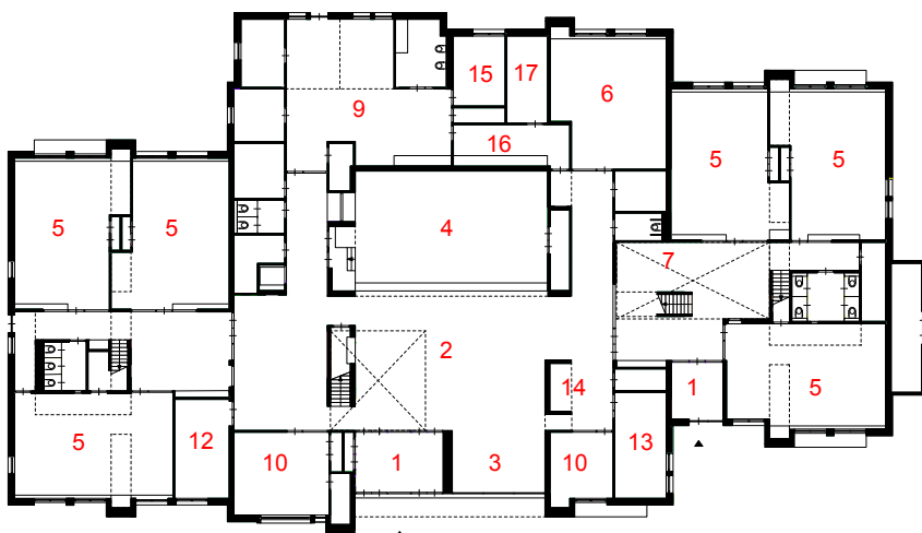
Begane grond
